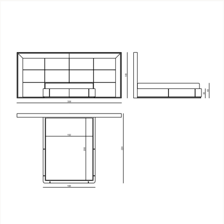
AUB152 L 338 x H 149 x W 227 cm
