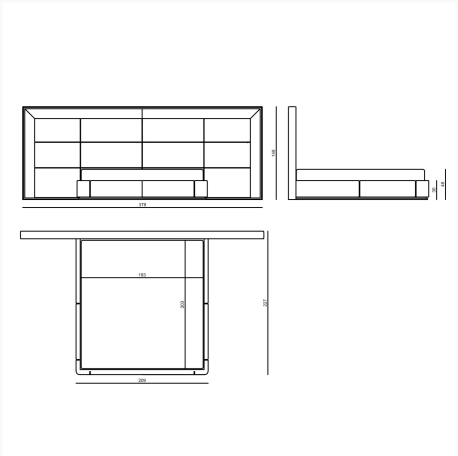
AUB193 L 379 x H 149 x W 227 cm
