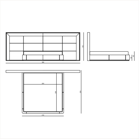
AUBL20 L 386 x H 149 x W 224 cm
