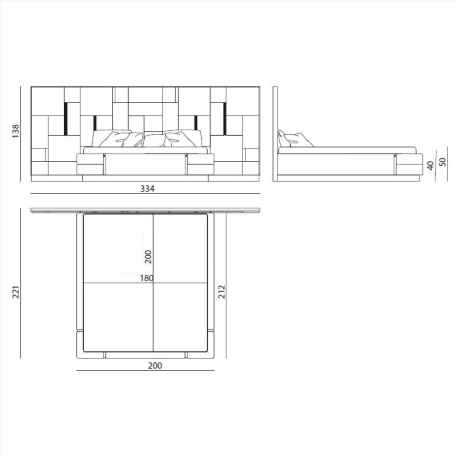
BLVL18 L 334 x H 138 x W 212 cm
