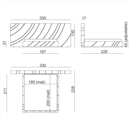
ULTL18 L 330 x H 130 x W 228 cm
