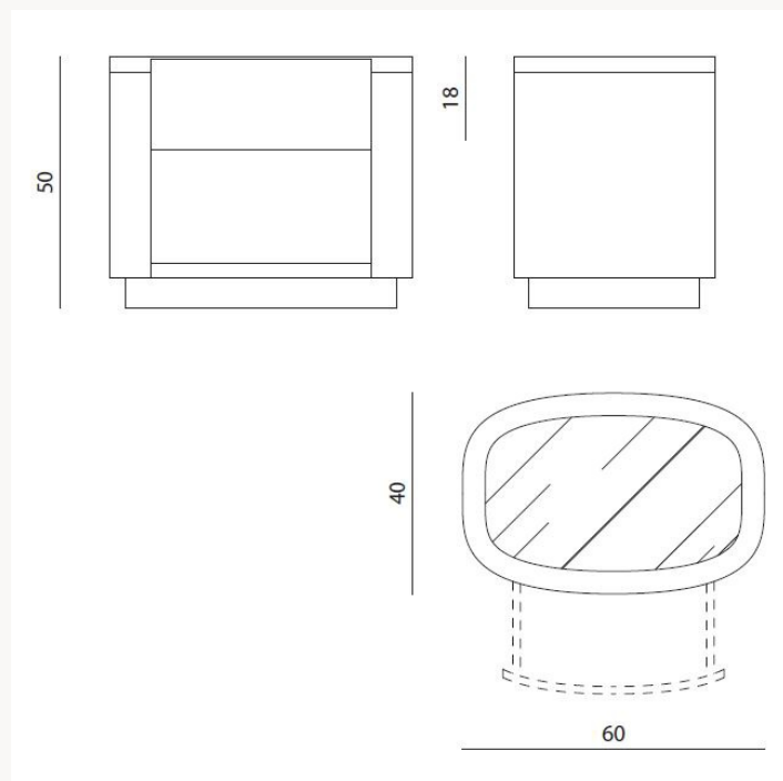
SKISKV L 60 x H 50 x W 40 cm
