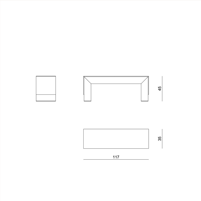
KLOKLB L 117 x H 45 x W 35 cm
