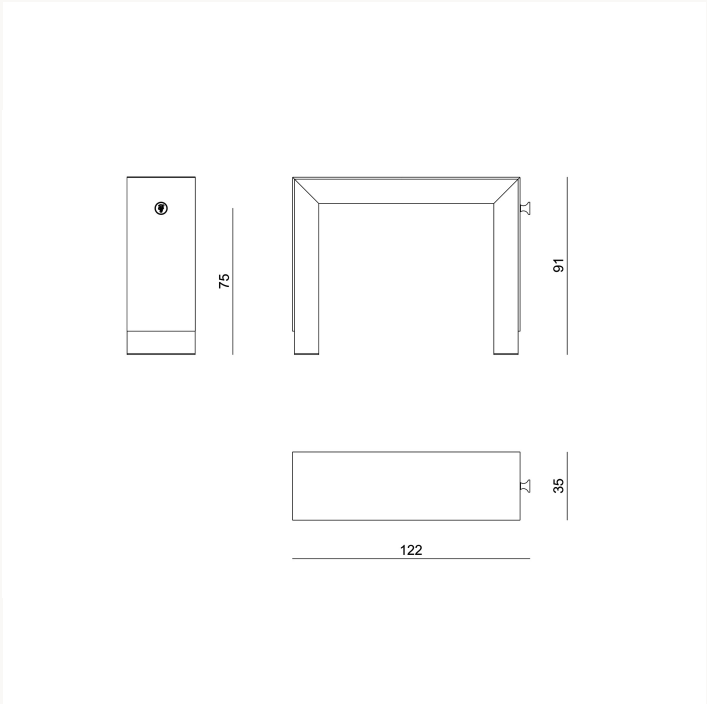
KLOKLC L 122 x H 91 x W 35 cm
