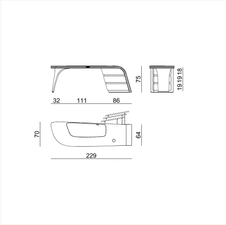
AMBJSX L 229 x H 75 x W 70 cm
