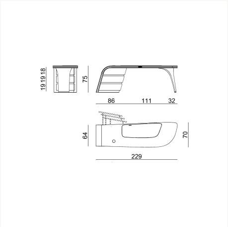
AMBJES L 229 x H 75 x W 70 cm
