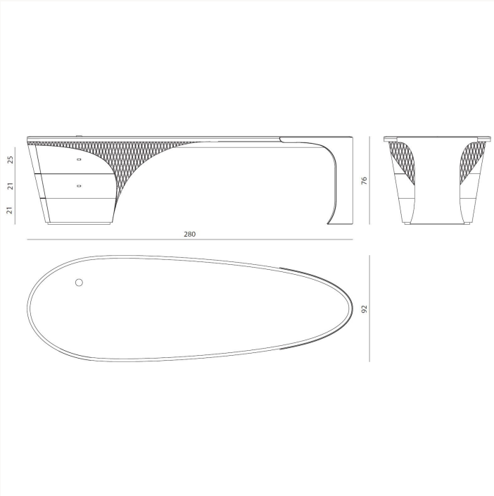
JET JES L 280 x H 76 x W 92 cm
