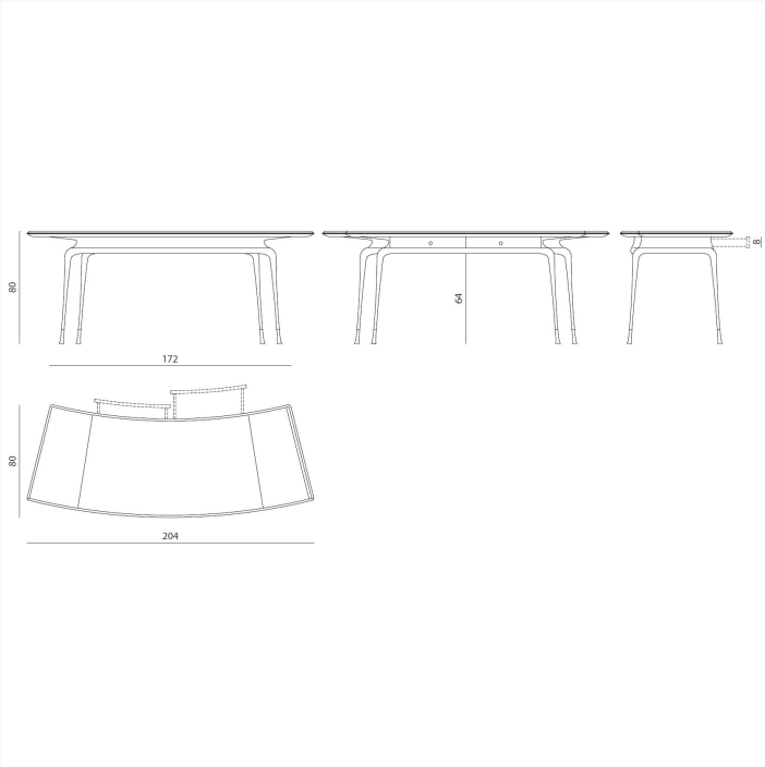
SNYW18 L 204 x H 80 x W 80 cm
