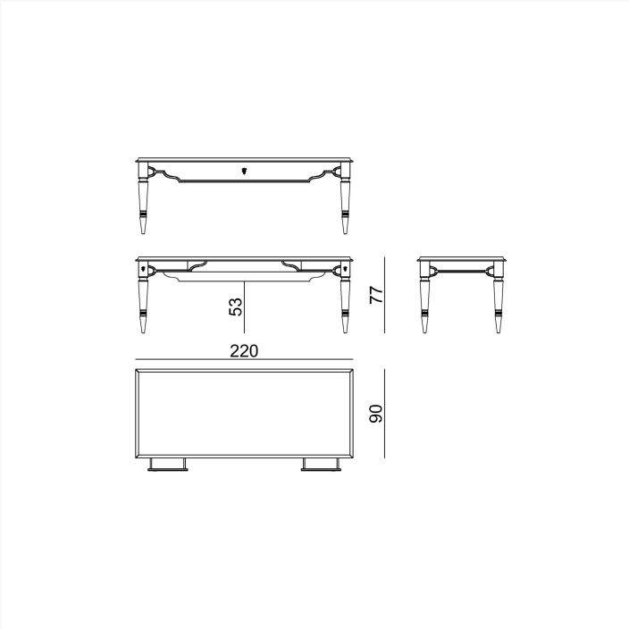
WIDWL2 L 220 x H 77 x W 90 cm
