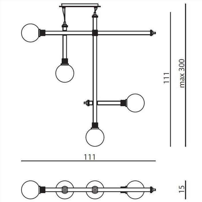
ALPLPQ L 111 x H 111 x W 15 cm
