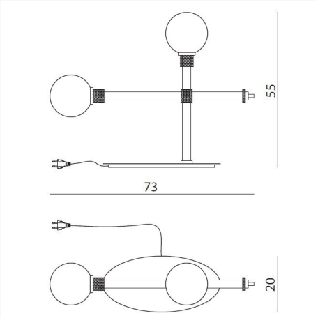
ALPBGG L 73 x H 55 x W 20 cm
