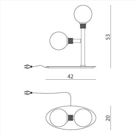
ALPBGF L 42 x H 53 x W 20 cm
