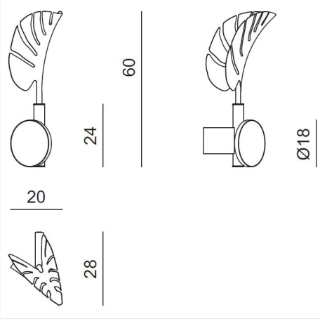
CIABG6 L 20 x H 60 x W 28 cm
