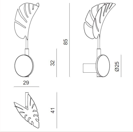
CIABG8 L 29 x H 85 x W 41 cm
