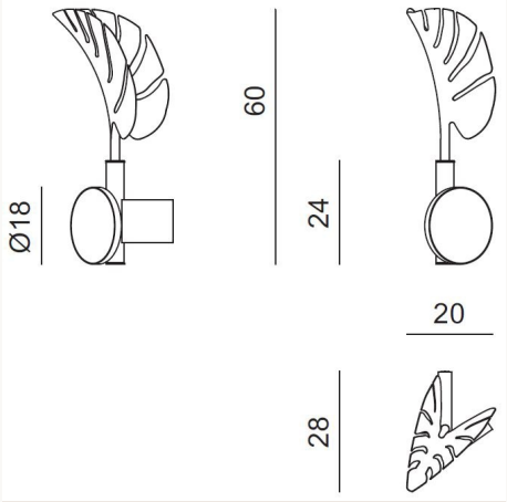
CIABG5 L 20 x H 60 x W 28 cm
