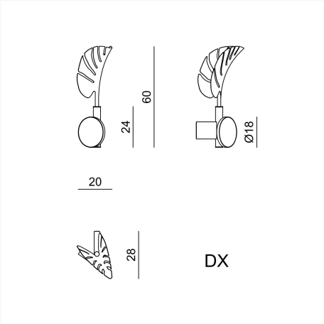
CIABG3 L 20 x H 60 x W 28 cm
