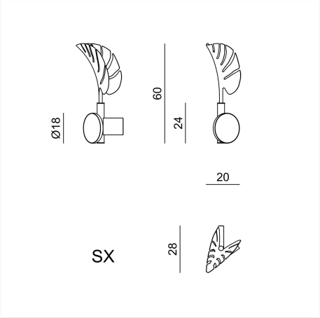
CIABG4 L 20 x W 28 cm
