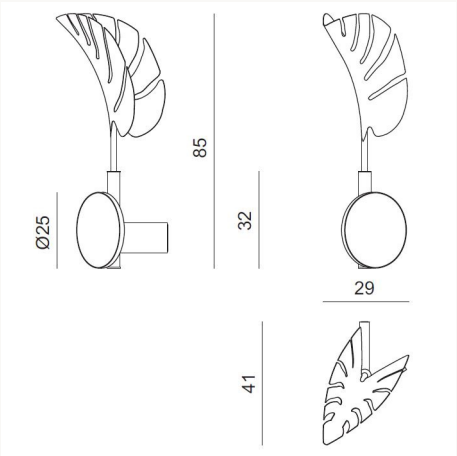
CIABG1 L 29 x H 85 x W 41 cm
