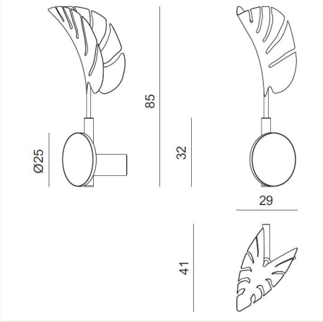
CIABG9 L 29 x H 85 x W 41 cm
