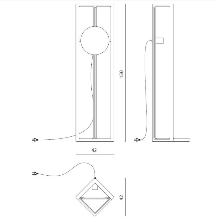
MOEBGB L 42 x H 150 x W 42 cm
