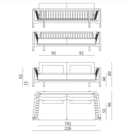
GRLD26 L 226 x H 80 x W 96 cm
