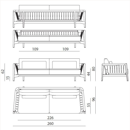
GRL260 L 260 x H 80 x W 96 cm
