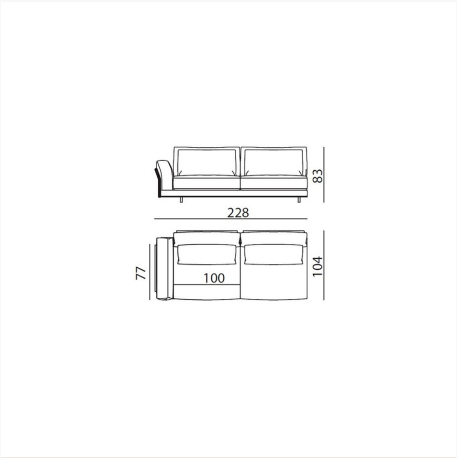
ANHE6B L 228 x H 83 x W104 cm
