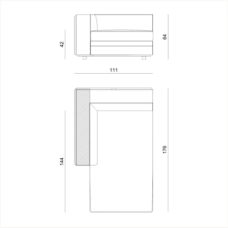
BYRK5I L 176 x H 64 x W 111 cm
