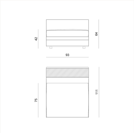
BYRK1L L 93 x H 64 x W 111 cm
