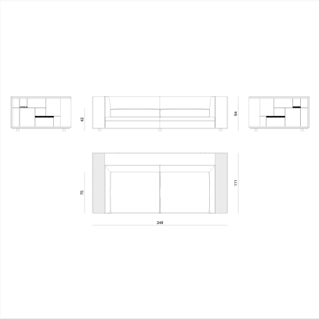
BYRK91 L 248 x H 64 x W 111 cm
