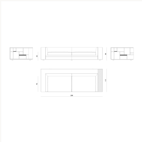
BYRK69 L 298 x H 64 x W 111 cm
