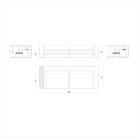
BYRK64 L 298 x H 64 x W 111 cm
