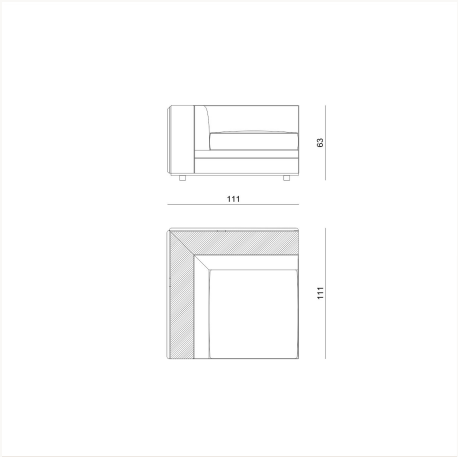
BYRK26 L 111 x H 64 x W 111 cm
