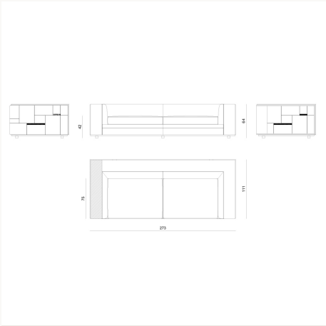
BYRK77 L 273 x H 64 x W 111 cm
