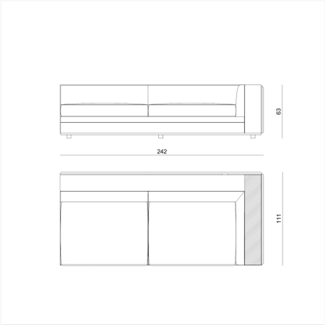
BYRK33 L 242 x H 64 x W 111 cm
