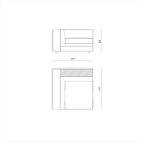
BYRK6H L 111 x H 64 x W 111 cm
