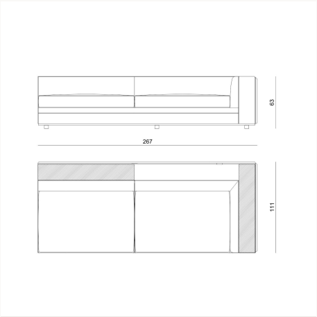
BYRK5E L 267 x H 64 x W 111 cm
