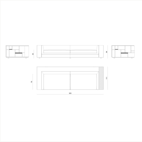
BYRK55 L 323 x H 64 x W 111 cm
