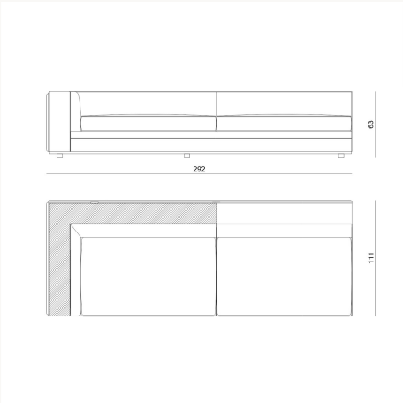
BYRK5D L 292 x H 64 x W 111 cm
