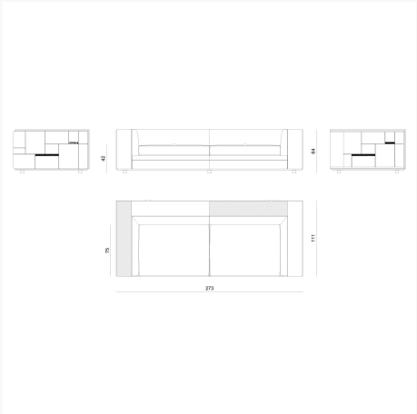
BYRK84 L 273 x H 64 x W 111 cm
