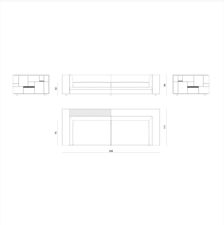
BYRK67 L 298 x H 64 x W 111 cm
