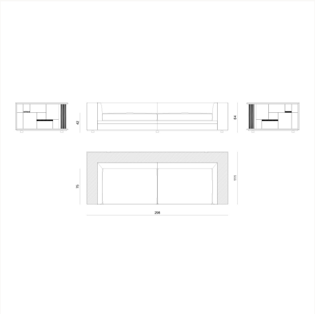
BYRK35 L 298 x H 64 x W 111 cm
