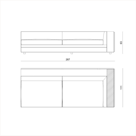
BYRK4E L 267 x H 64 x W 111 cm
