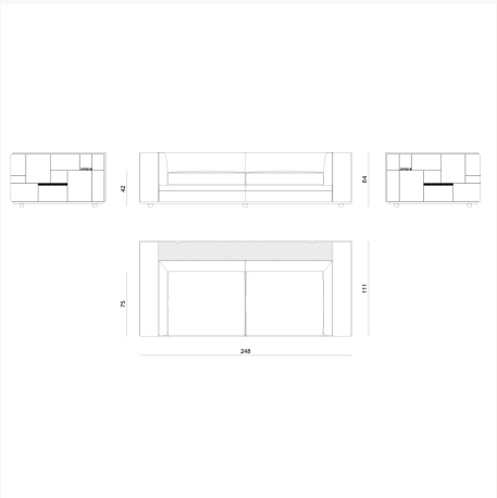
BYRK28 L 248 x H 64 x W 111 cm
