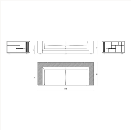
BYRK36 L 273 x H 64 x W 111 cm
