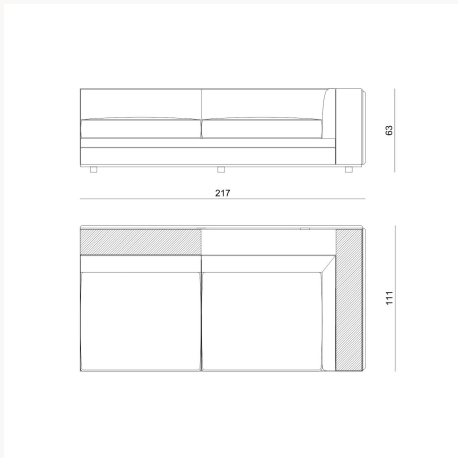
BYRK9F L 217 x H 64 x W 111 cm
