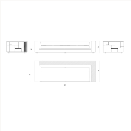
BYRK62 L 323 x H 64 x W 111 cm
