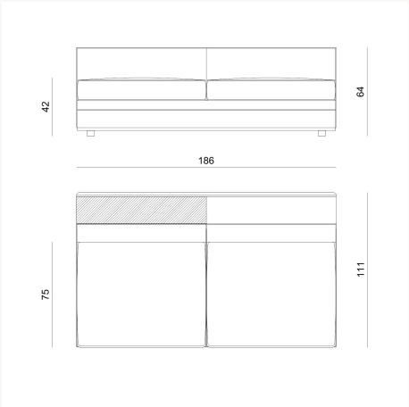
BYRK09 L 186 x H 64 x W 111 cm
