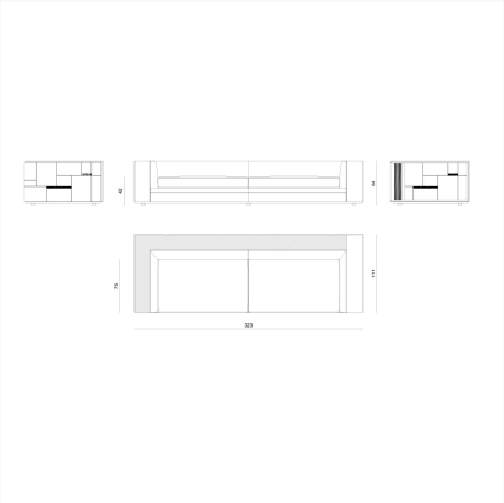
BYRK59 L 323 x H 64 x W 111 cm
