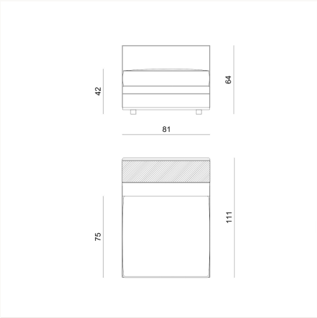
BYRK46 L 81 x H 64 x W 111 cm
