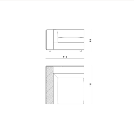
BYRK20 L 111 x H 64 x W 111 cm
