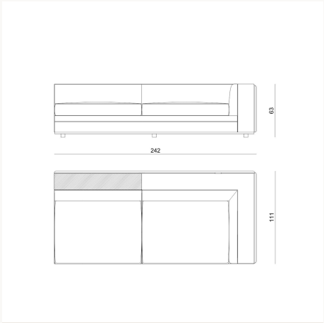
BYRK6G L 242 x H 64 x W 111 cm
