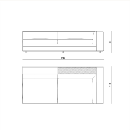
BYRK9G L 242 x H 64 x W 111 cm
