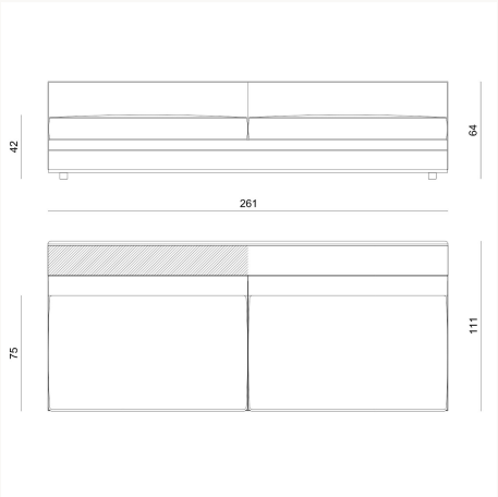
BYRK7D L 261 x H 64 x W 111 cm
