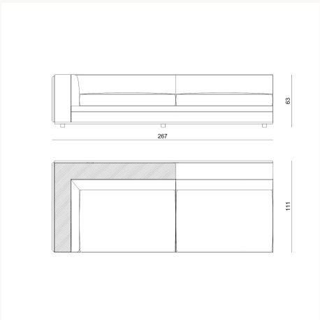
BYRK29 L 267 x H 64 x W 111 cm
