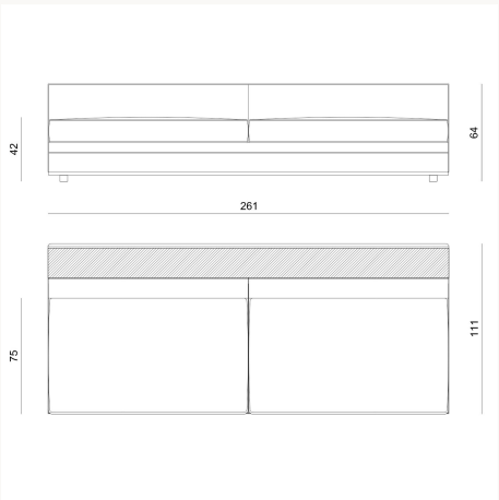
BYRK9D L 261 x H 64 x W 111 cm
