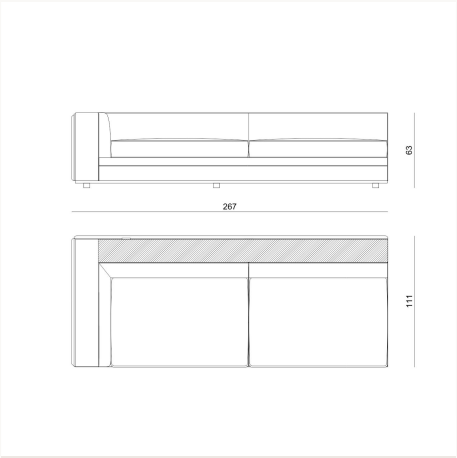
BYRK3E L 267 x H 64 x W 111 cm
