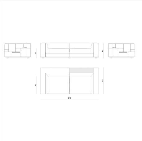
BYRK95 L 248 x H 64 x W 111 cm
