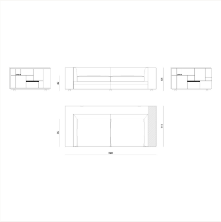
BYRK94 L 248 x H 64 x W 111 cm
