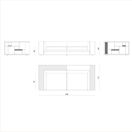
BYRK99 L 248 x H 64 x W 111 cm
