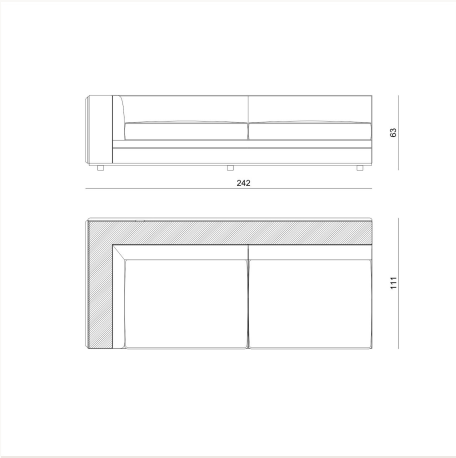
BYRK07 L 242 x H 64 x W 111 cm
