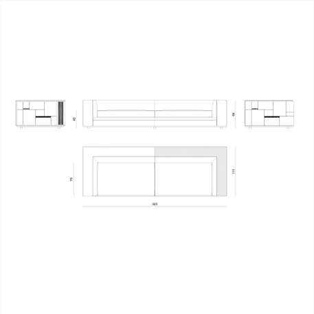
BYRK61 L 323 x H 64 x W 111 cm
