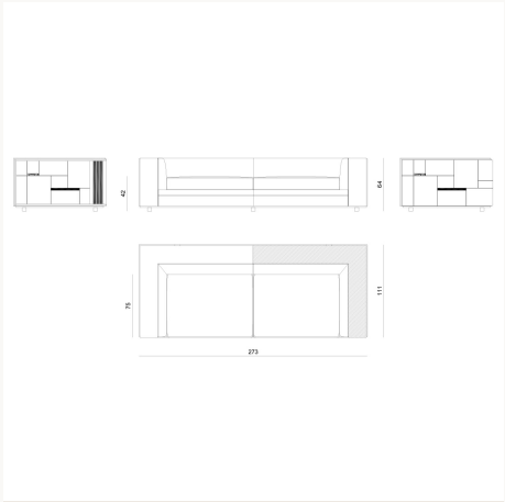
BYRK87 L 273 x H 64 x W 111 cm
