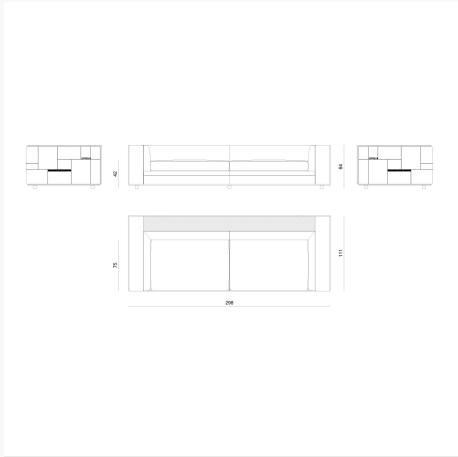
BYRK66 L 298 x H 64 x W 111 cm
