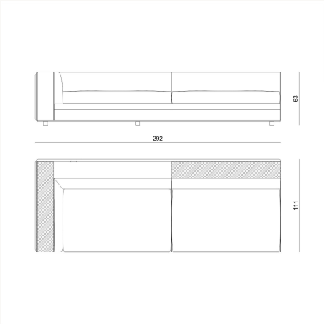
BYRK4C L 292 x H 64 x W 111 cm
