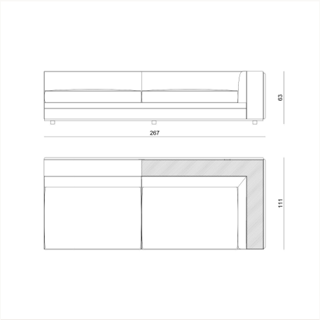
BYRK0E L 267 x H 64 x W 111 cm
