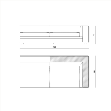
BYRK49 L 242 x H 64 x W 111 cm
