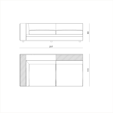
BYRK5F L 217 x H 64 x W 111 cm
