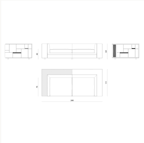
BYRK97 L 248 x H 64 x W 111 cm
