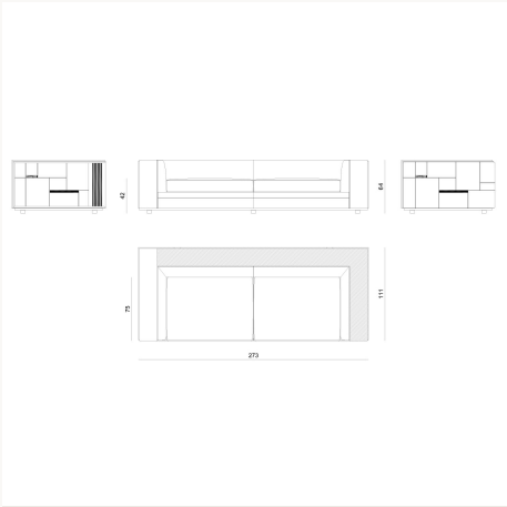
BYRK88 L 273 x H 64 x W 111 cm
