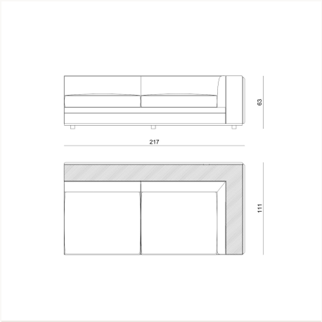
BYRK4H L 217 x H 64 x W 111 cm
