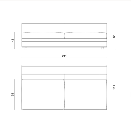
BYRK4F L 211 x H 64 x W 111 cm
