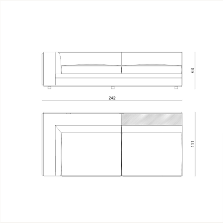
BYRK02 L 242 x H 64 x W 111 cm
