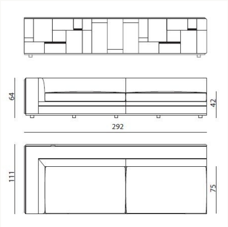
BABEM0 L 292 x H 64 x W 111 cm
