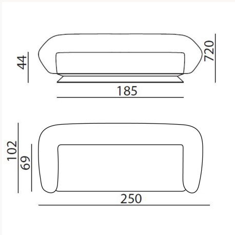
CTZD25 L 250 x H 72 x W102 cm
