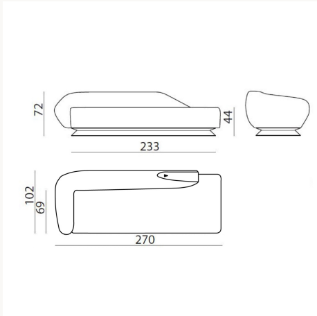
CTZ2SX L 270 x H 72 x W102 cm
