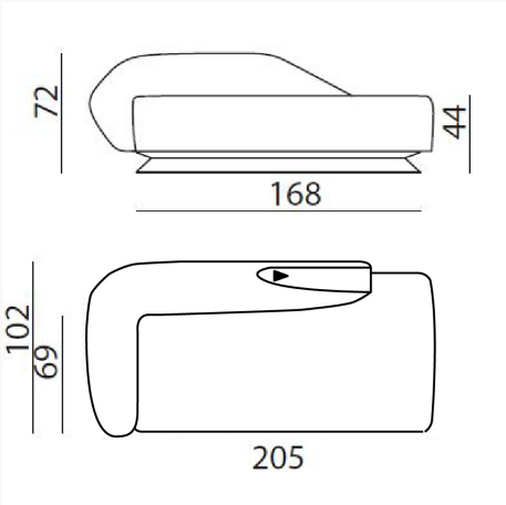
CTZE2S L 205 x H 72 x W102 cm
