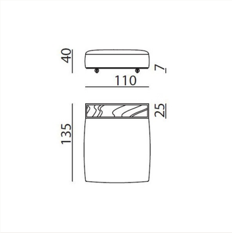
DS538P L 110 x H 40 x W 135 cm
