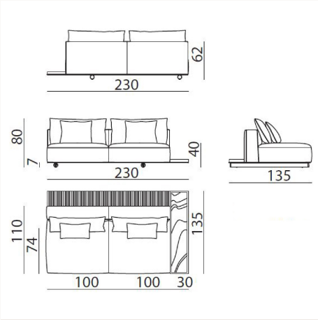
DS527P L 230 x H 80 x W 135 cm
