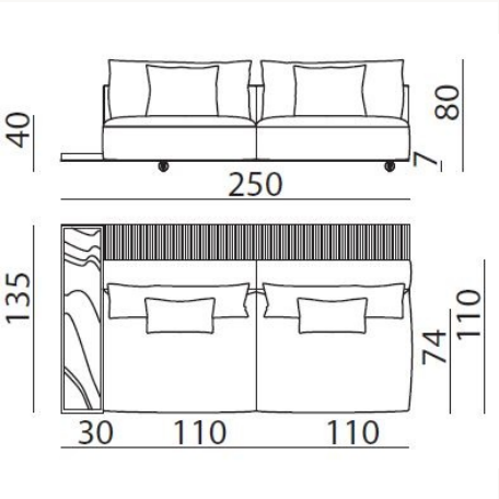
DS532P L 250 x H 80 x W 135 cm
