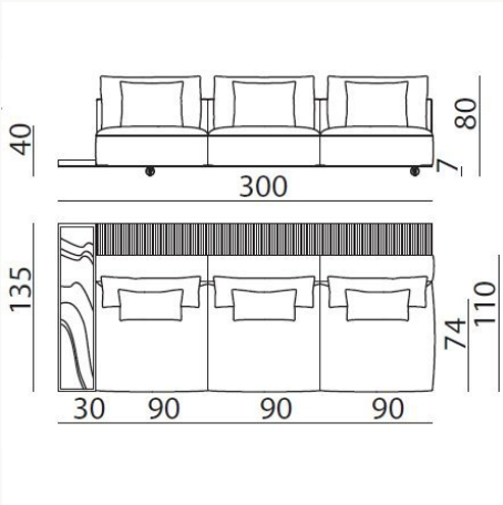
DS534P L 300 x H 80 x W 135 cm
