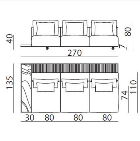
DS533P L 270 x H 80 x W 135 cm
