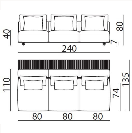
DS525P L 240 x H 80 x W 135 cm
