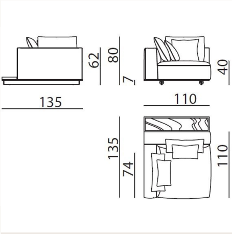
DS5Q36 L 110 x H 80 x W 135 cm
