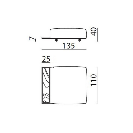
DS537P L 135 x H 40 x W 110 cm
