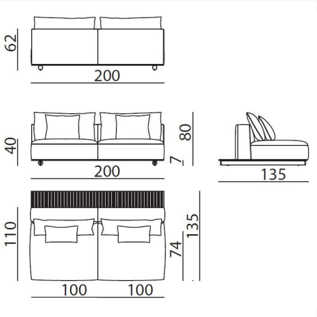
DS523P L 200 x H 80 x W 135 cm
