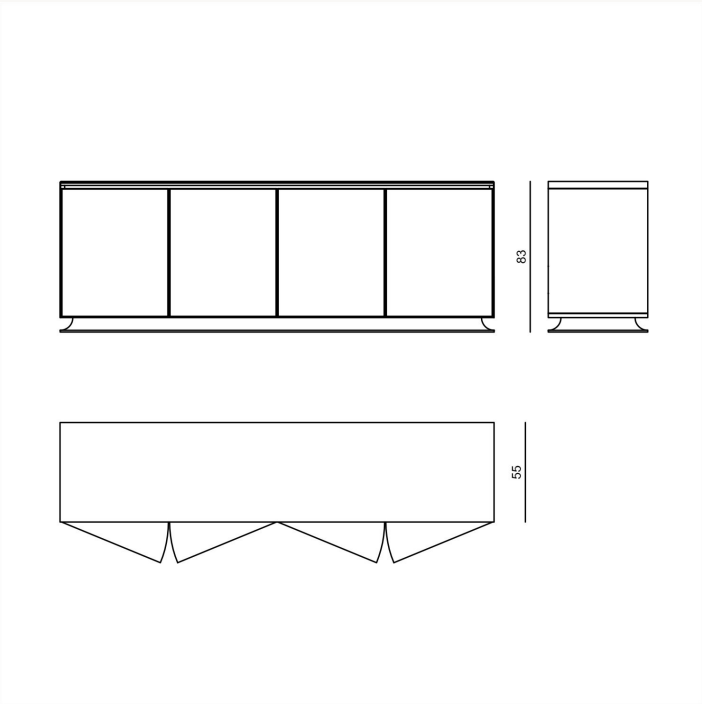
AUOAO6 L 240 x H 84 x W 55 cm
