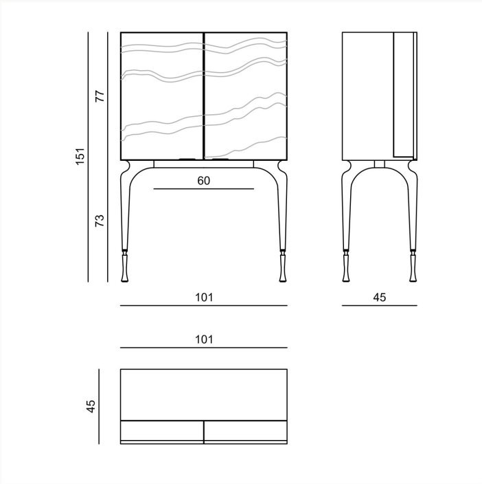
AUOAO3 L 101 x H 151 x W 45 cm
