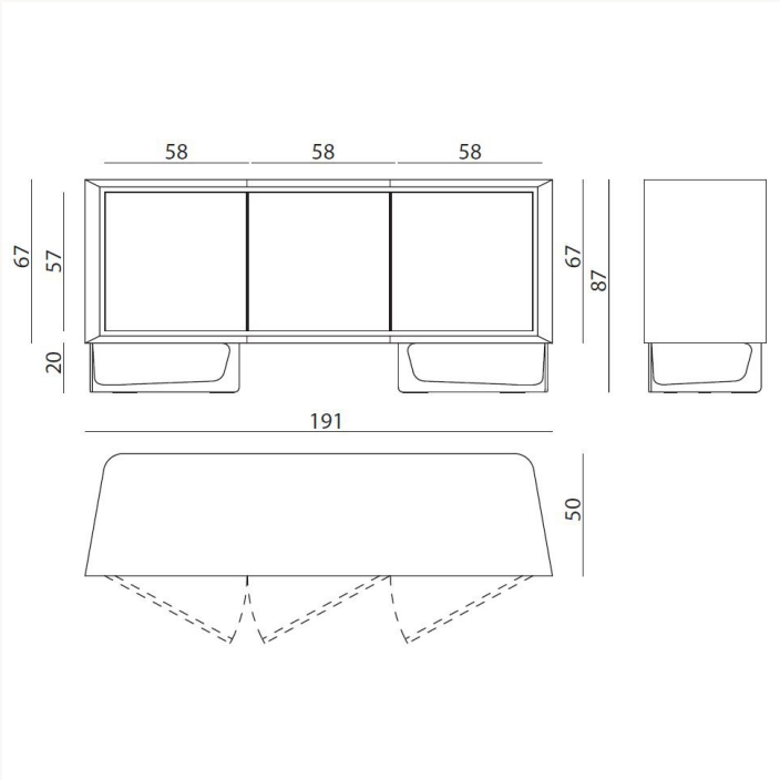
AZIMBN L 191 x H 87 x W 50 cm
