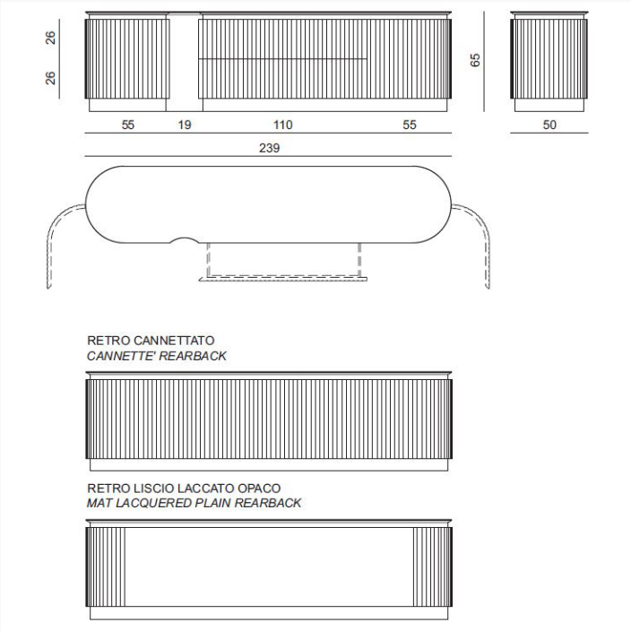
LNRB2A L 240 x H 65 x W 50 cm
