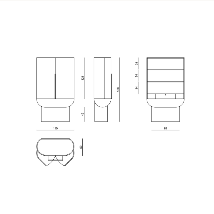
SIO SM2 L 110 x H 188 x W 50 cm
