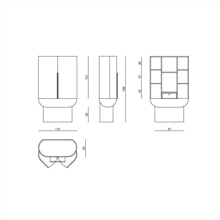
SIO SM3 L 110 x H 188 x W 50 cm
