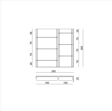
TIVPRA L 262 x H 265 x W 25 cm
