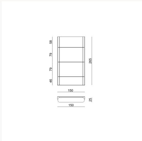
TIVTIV L 150 x H 265 x W 25 cm
