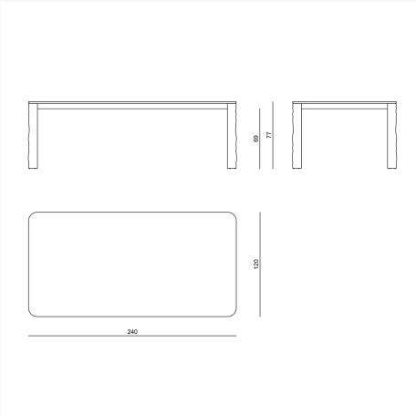
SRMVT0 L 240 x H 77 x W 120 cm
