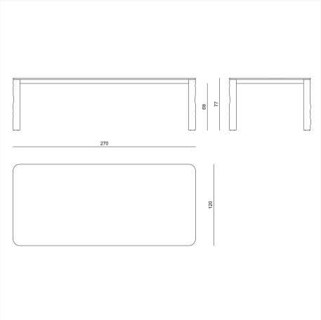
SRMKR8 L 270 x H 77 x W 120 cm
